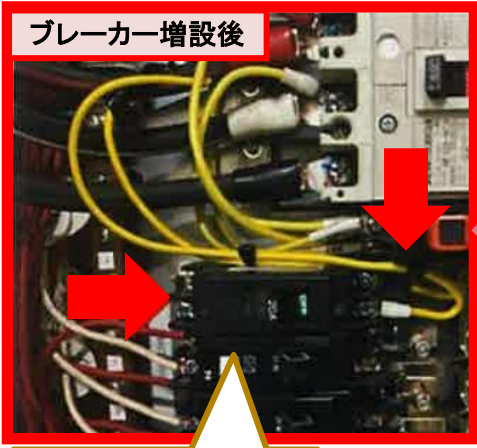
ブレーカー増設及び 1次側に配線
