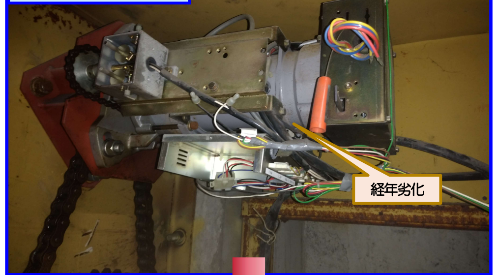
工事前(既存開閉機)
