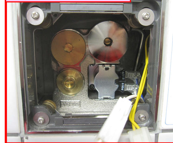
工事後 (フラッシュバルブ取替)
