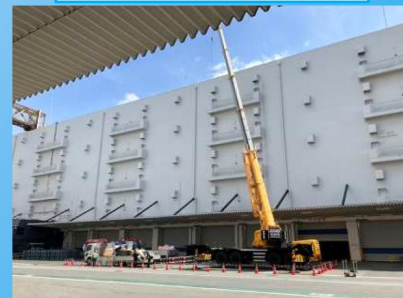
エレベーター準撤去更新工事 クレーン揚重作業状況
