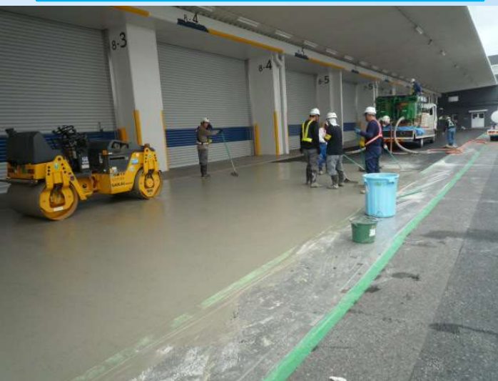
低床倉庫前 舗装更新施工状況
