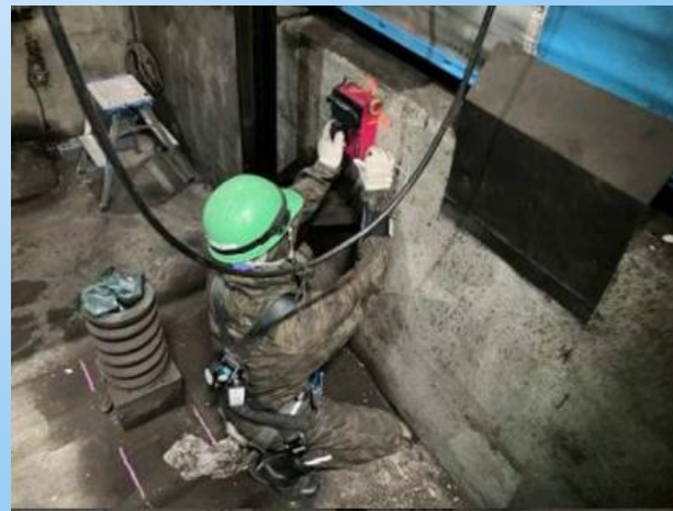
エレベーター準撤去更新工事状況 ピット内埋設探査
