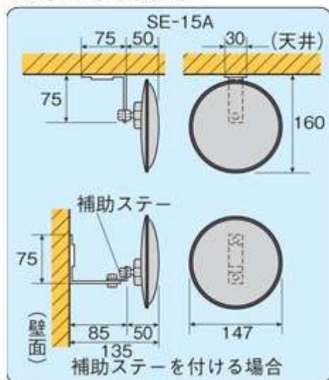
SE-15BA 取り付け図・構造図
